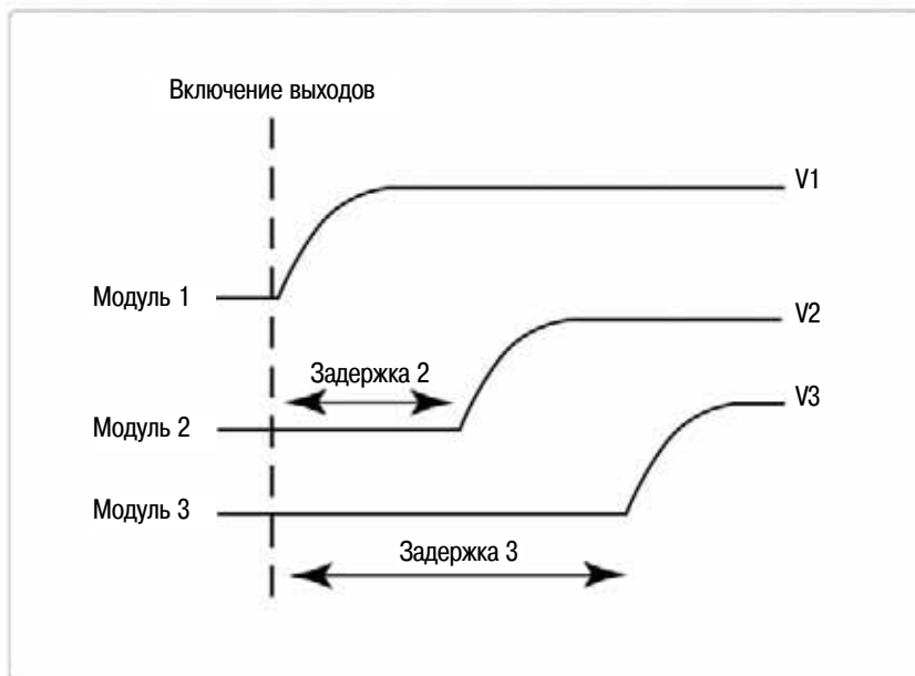
Рисунок 2 - Последовательность включения выходов
